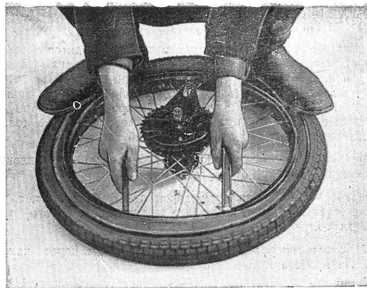
Рис. 32б. Одевание покрышки на колесо.
