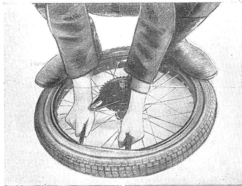
Рис. 31. Снятие покрышки с колеса.
