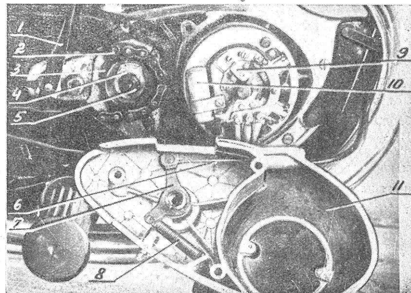
Рис. 11. Правая часть картера (со снятой крышкой).
