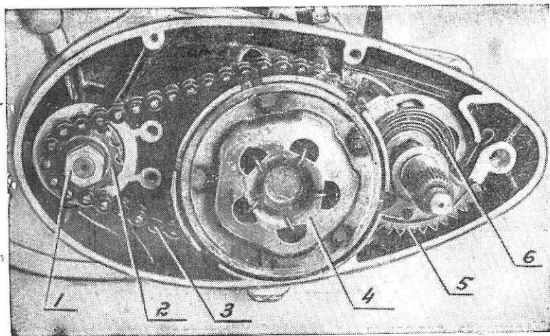
Рис. 10. Передняя передача и сцепление.
