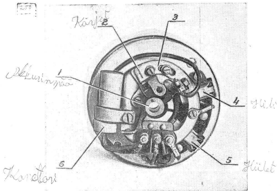
Рис. 23. Генератор со стороны крышки.
