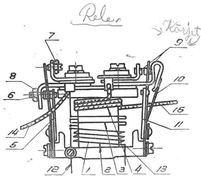
Рис. 26. Реле-регулятор.
