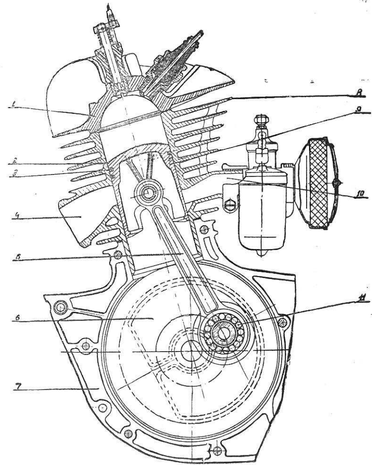
Рис. 6 Двигатель. (Продольный разрез).
