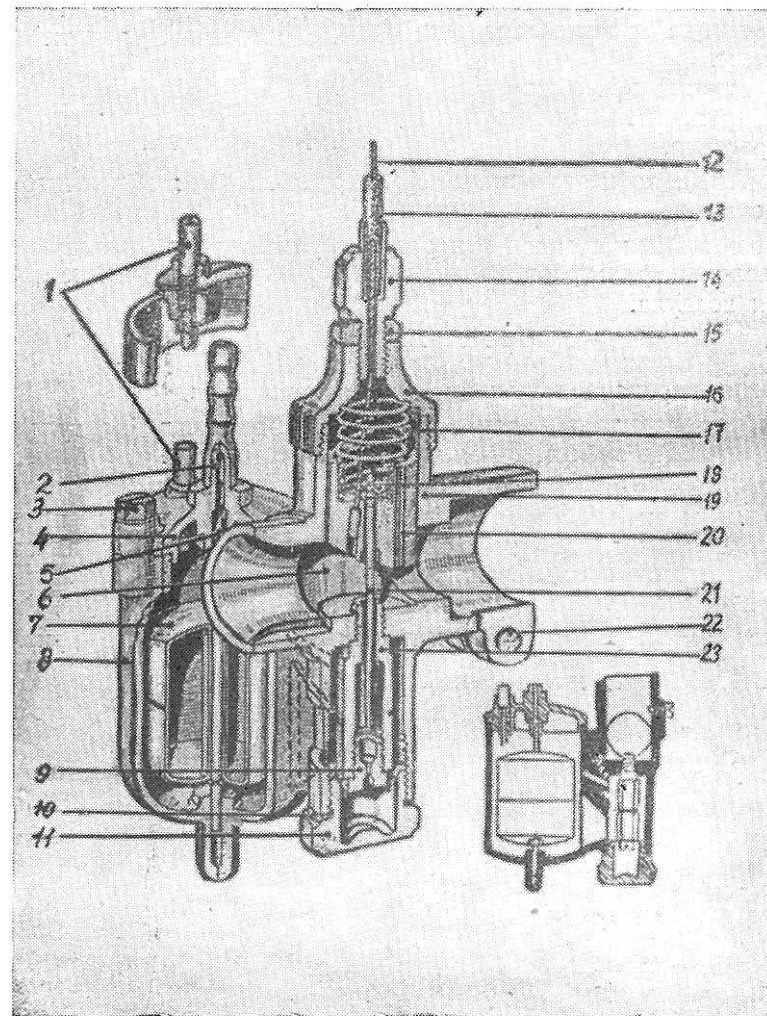
Рис. 9. Карбюратор К—30. р(азрез)
