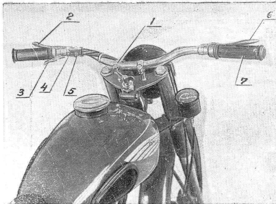
Рис. 20. Рулевое управление
