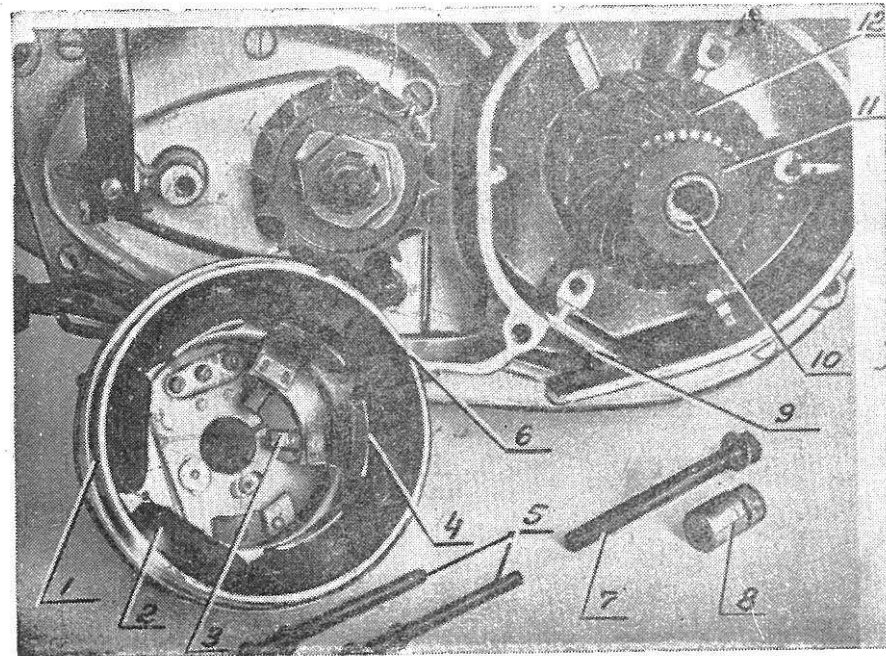
Рис. 22. Генератор в разобранном виде.
