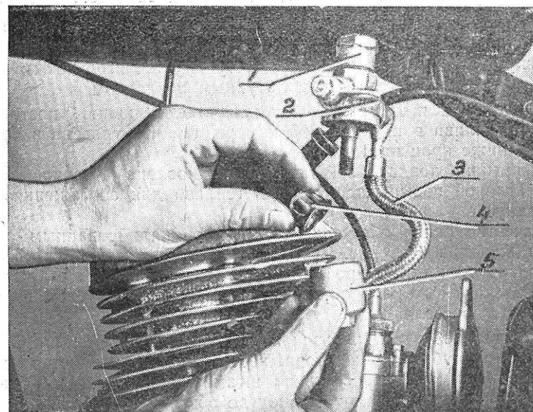
Рис. 8. Чистка отстойника.
