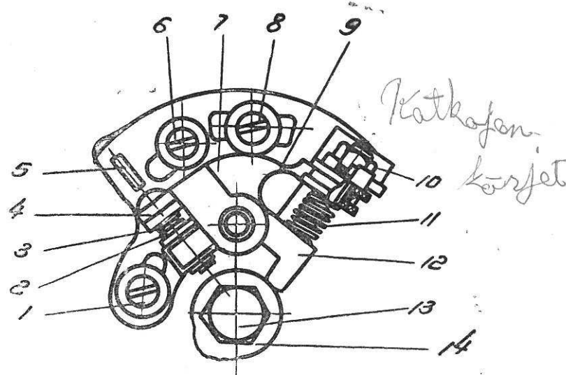
Рис. 24. Прерыватель
