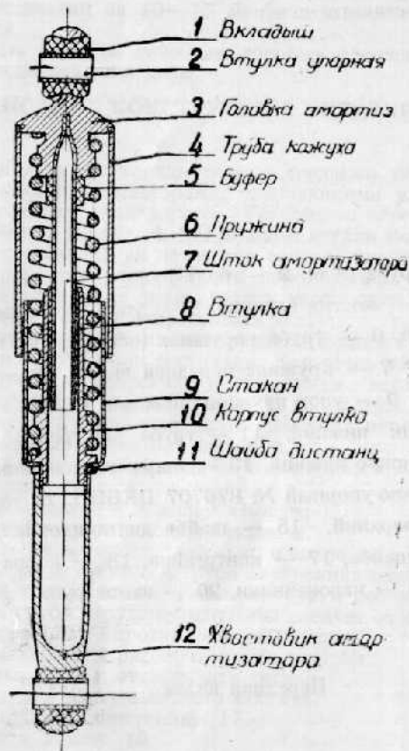
Рис. 5. Амортизатор задней подвески.
